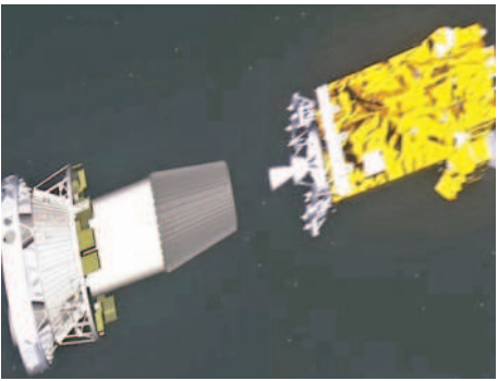
అంతరిక్షంలో సూర్యుని వైపు దూసుకుపోతూ రాకెట్ నుంచి విడిపోయిన ఆదిత్య ఎల్1
